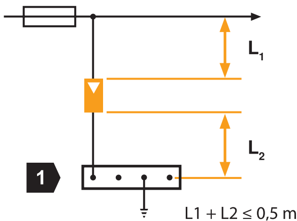
Maximální délka přívodu podle normy ČSN 33 2000-5-534 (IEC 60364-5-53)
