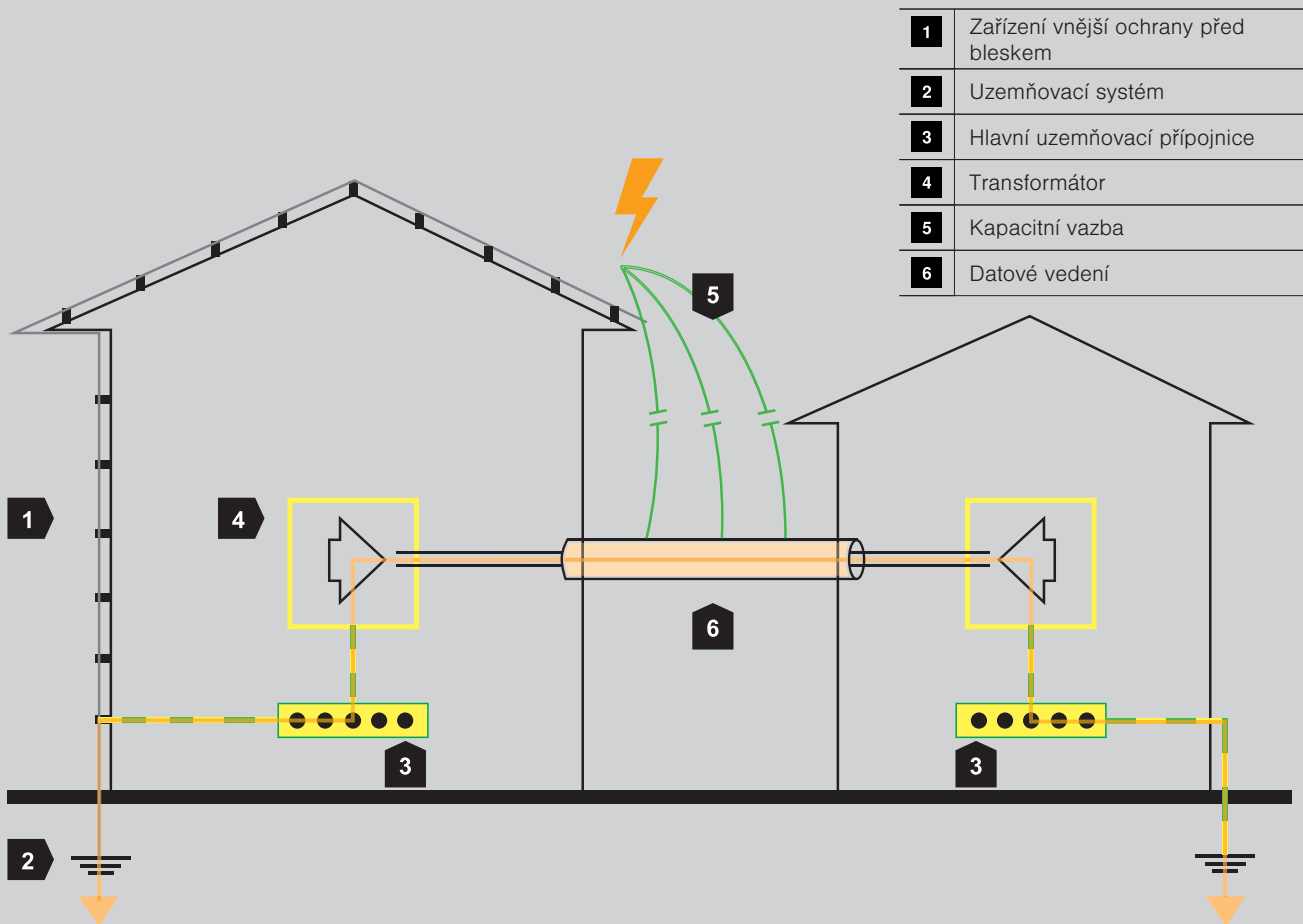
Kapacitní vazba při přímém úderu blesku
