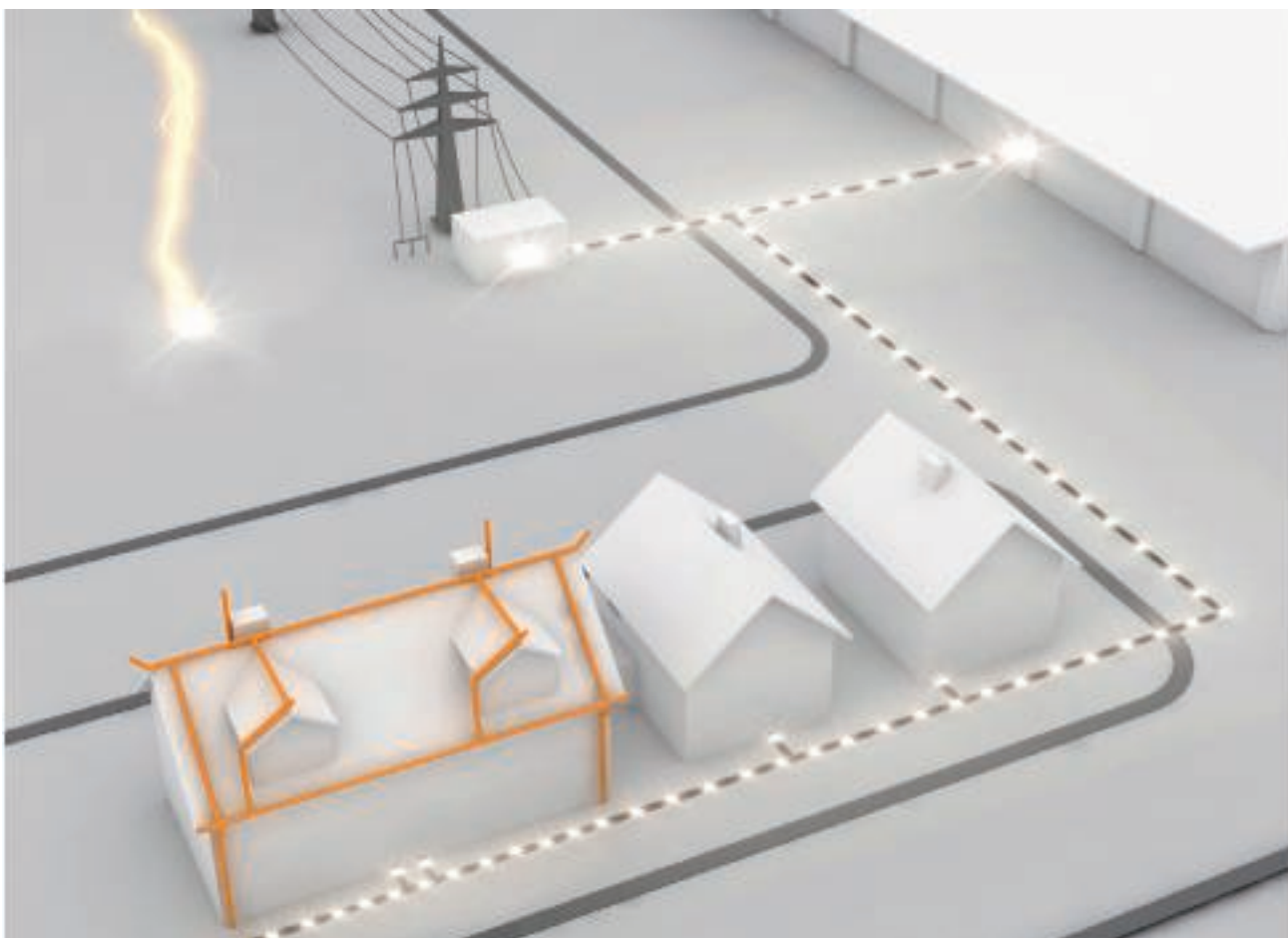
Ohrožení galvanicky zavádným přepětím přenášeným po vedení
