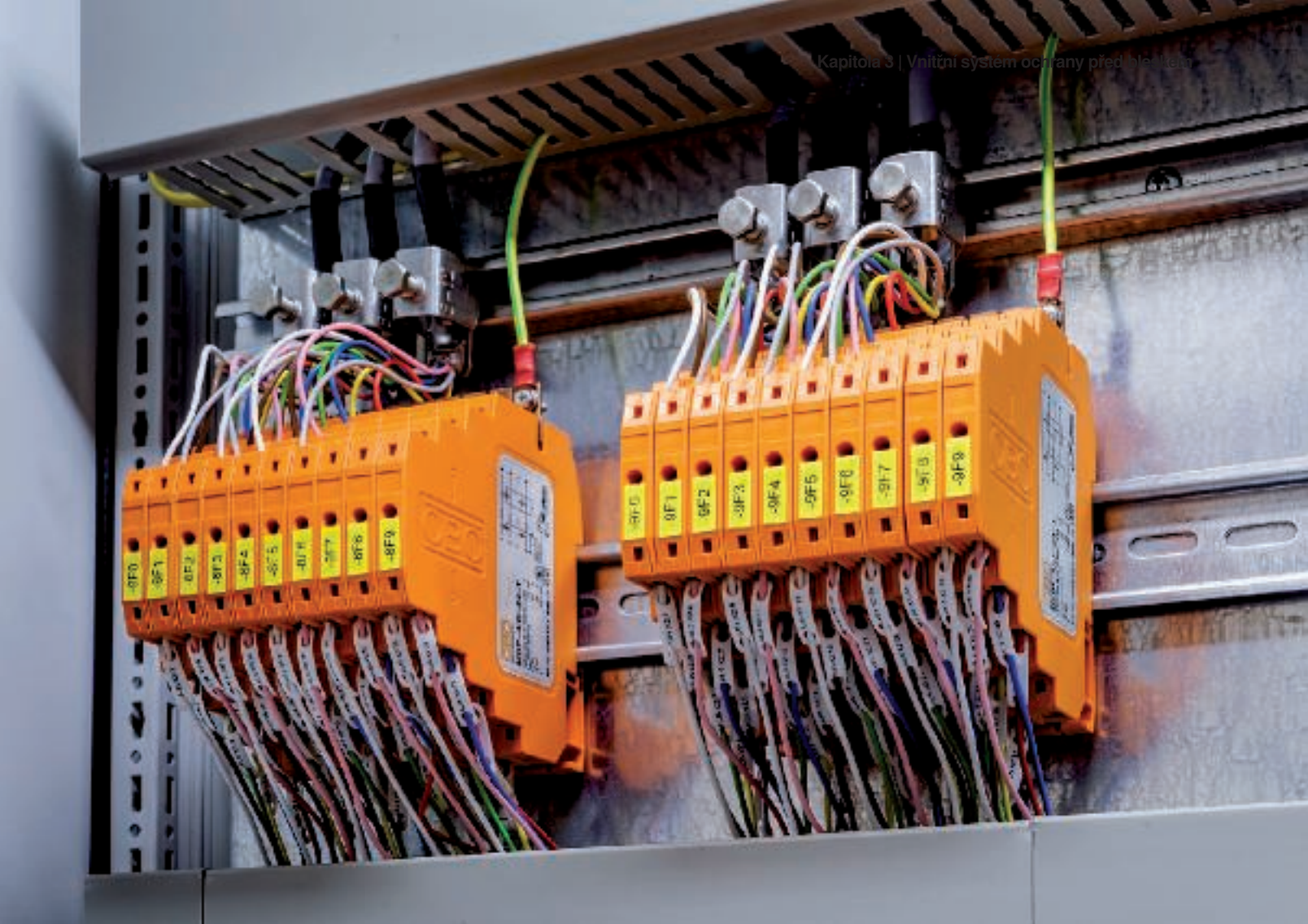
Instalace svodiče bleskových proudů MDP ve skříňovém rozvaděči
