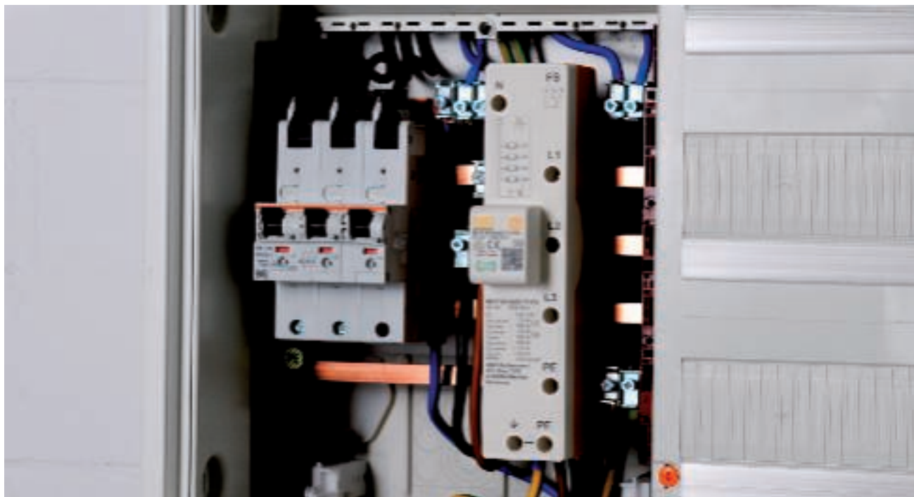
Kombinovaný svodič typu 1 + 2 MCF...NAR na 40 mm sběrné liště v přípojovacím prostoru na straně sítě
