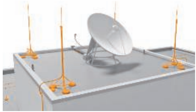
Oddělená ochrana před bleskem s jímacími tyčemi
