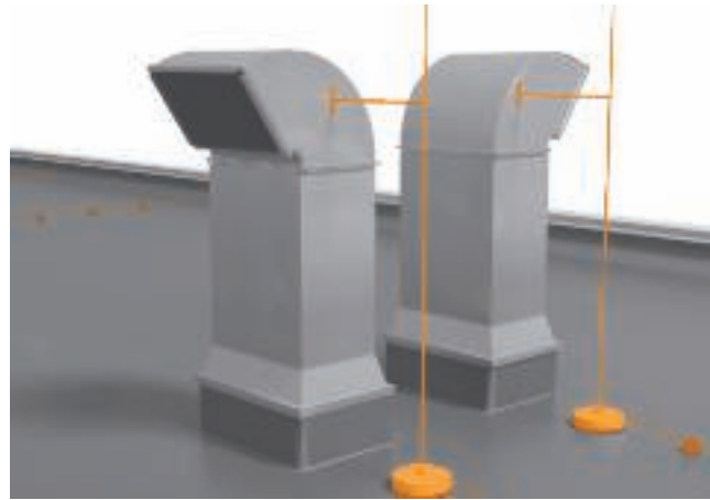
Jímací stožár s nastavitelným izolačním příčnickem
