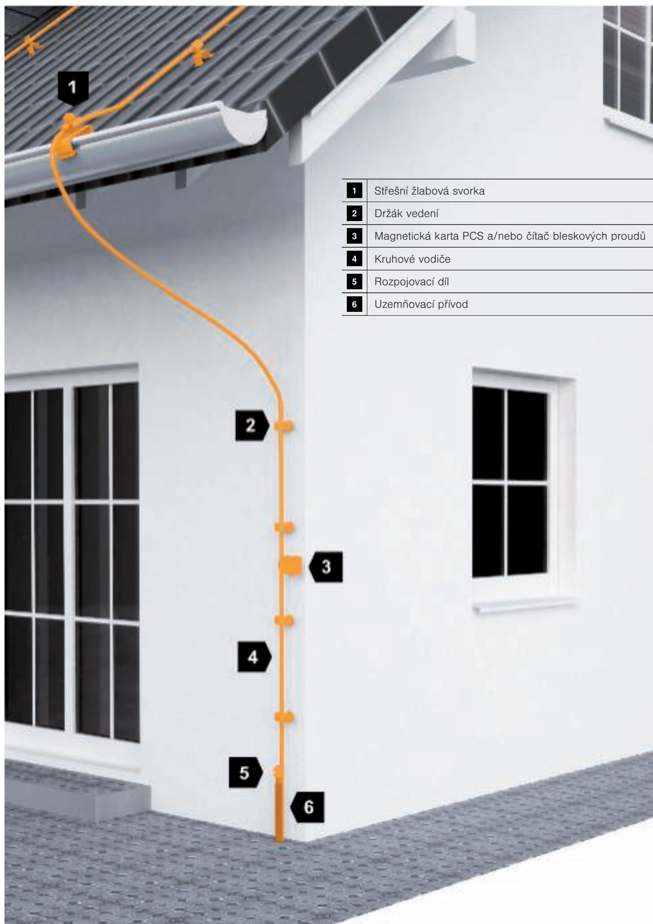
Princip instalace - svodová zařízení
