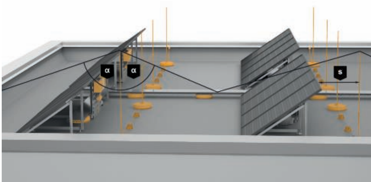
Ochranný úhel a oddělovací vzdálenost jímacích tyčí na fotovoltaickém zařízení
