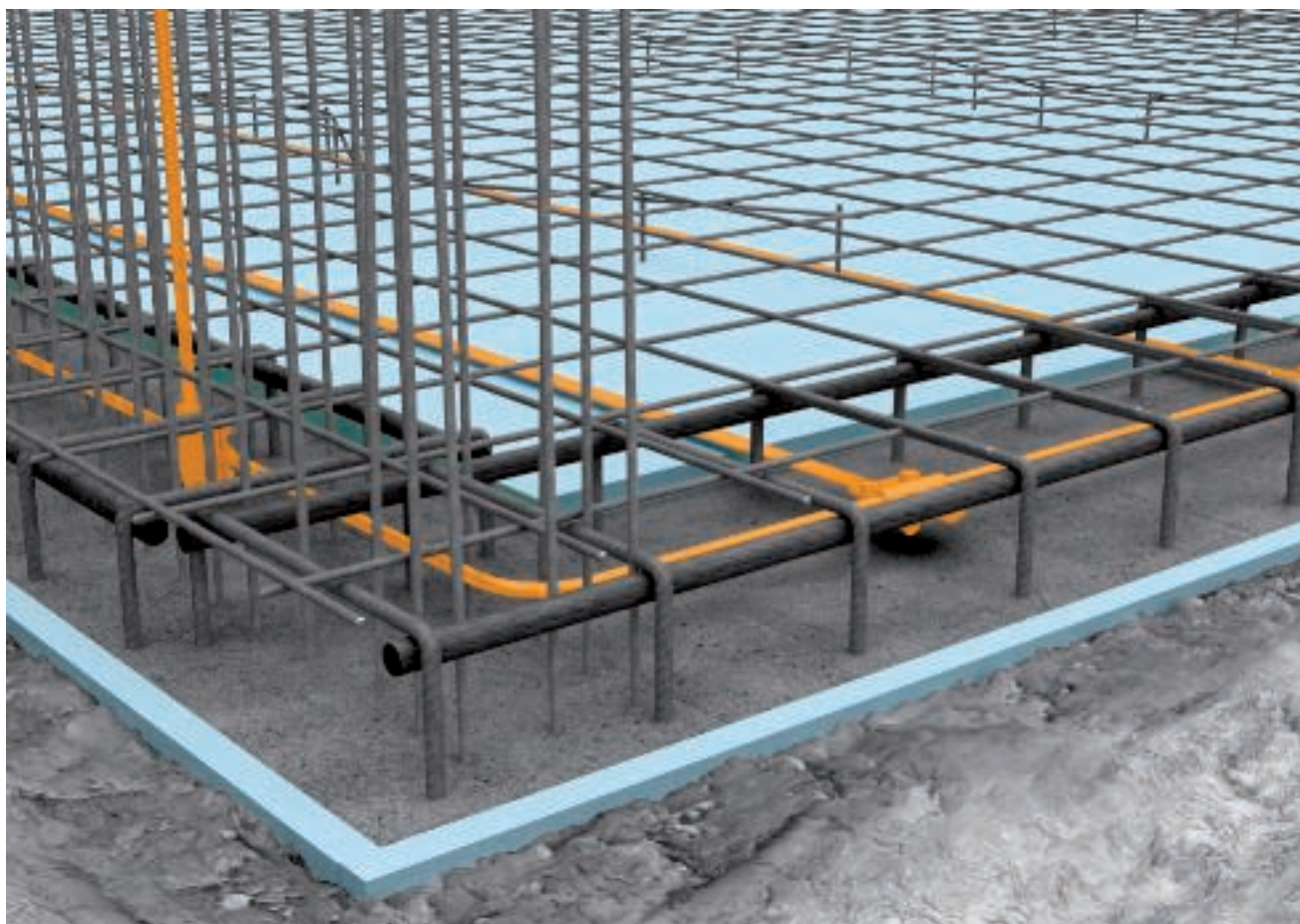
Izolovaná podlahová deska (obvodová izolace, zde: modrá)
