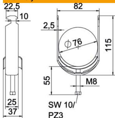
Rozměry
